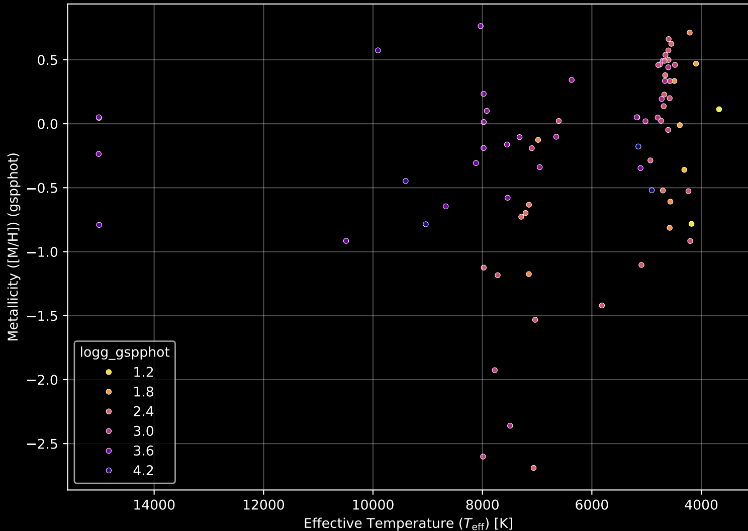
APOGEE DR17 Field: [317+00] Stellar Population Parameters (n= 77)
